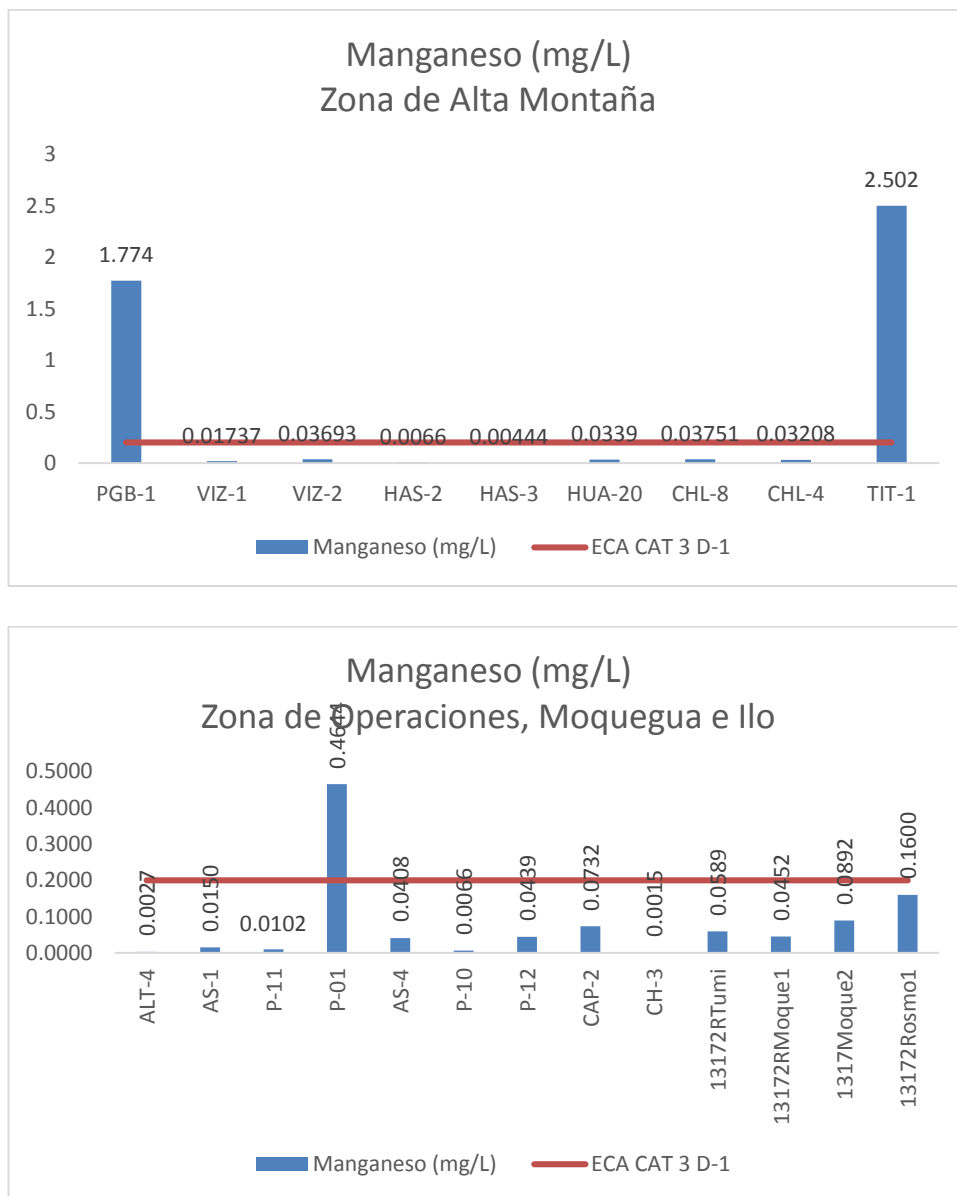
Gráfico 29. Variación espacial del contenido de manganeso en las estaciones de monitoreo de calidad de agua superficial - zona de alta montaña, zona de operaciones, Moquegua e Ilo del MAP-5 setiembre 2017.
