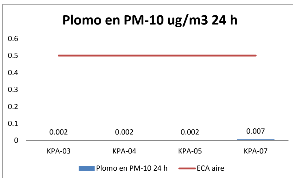
Gráfico 40. Variación espacial del contenido de plomo en material particulado menor a 10 \mu\text{m} de las diferentes estaciones de monitoreo de calidad de aire del MAP-5 setiembre 2017.
