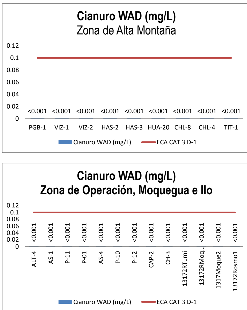
Gráfico 08. Variación espacial del contenido de cianuro de las diferentes estaciones de monitoreo de calidad de agua superficial – zona de alta montaña, zona de operaciones, Moquegua e Ilo del MAP-5 setiembre 2017.
