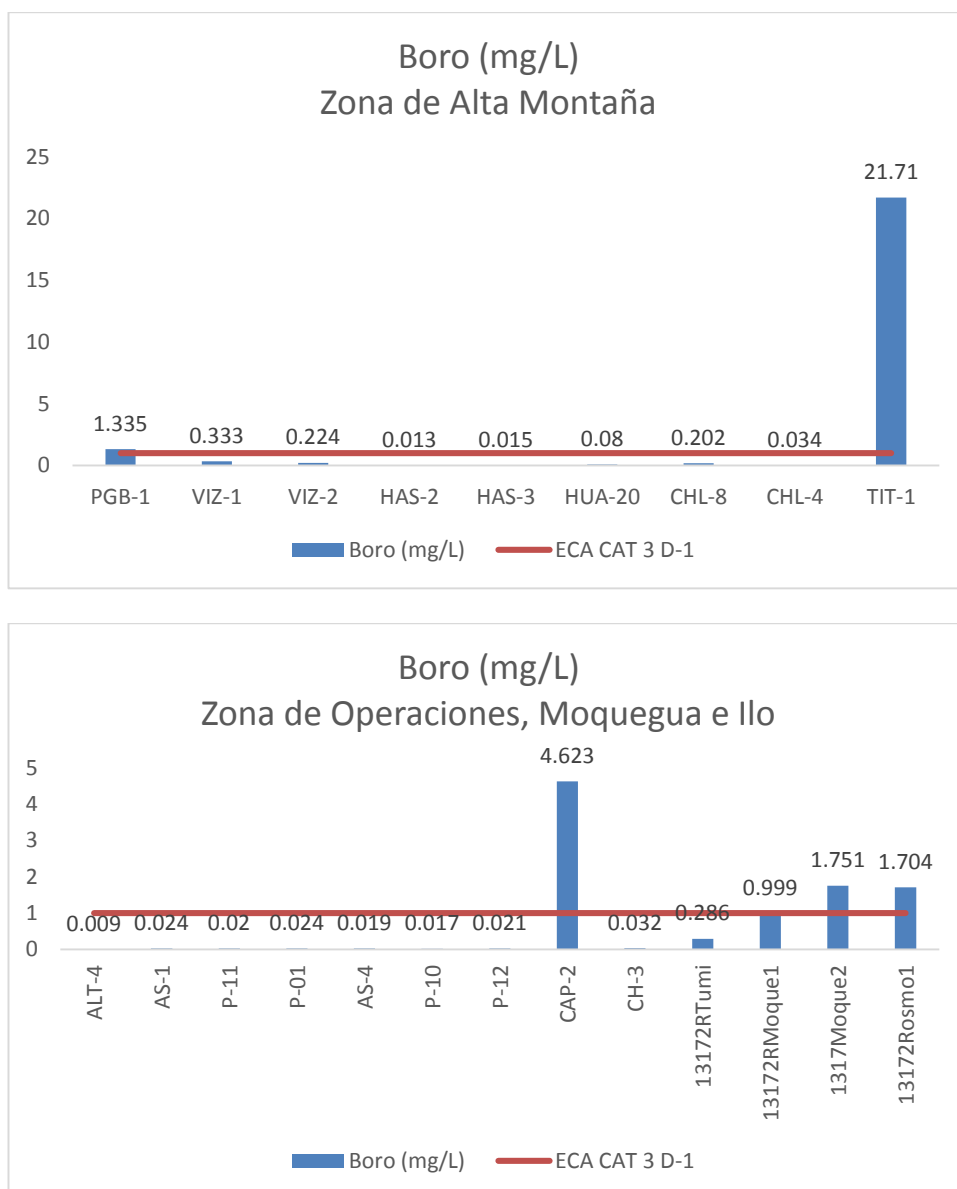
Gráfico 23. Variación espacial del contenido de boro en las estaciones de monitoreo de calidad de agua superficial – zona de alta montaña, zona de operaciones, Moquegua e Ilo del MAP-5 setiembre 2017.
