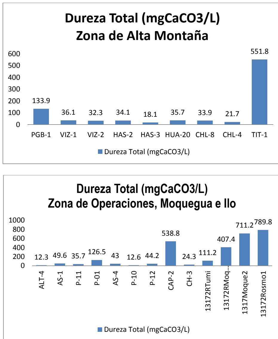
Gráfico 11. Variación espacial del valor de la dureza de las diferentes estaciones de monitoreo de calidad de agua superficial – zona de alta montaña, zona de operaciones, Moquegua e Ilo del MAP-5 setiembre 2017.
