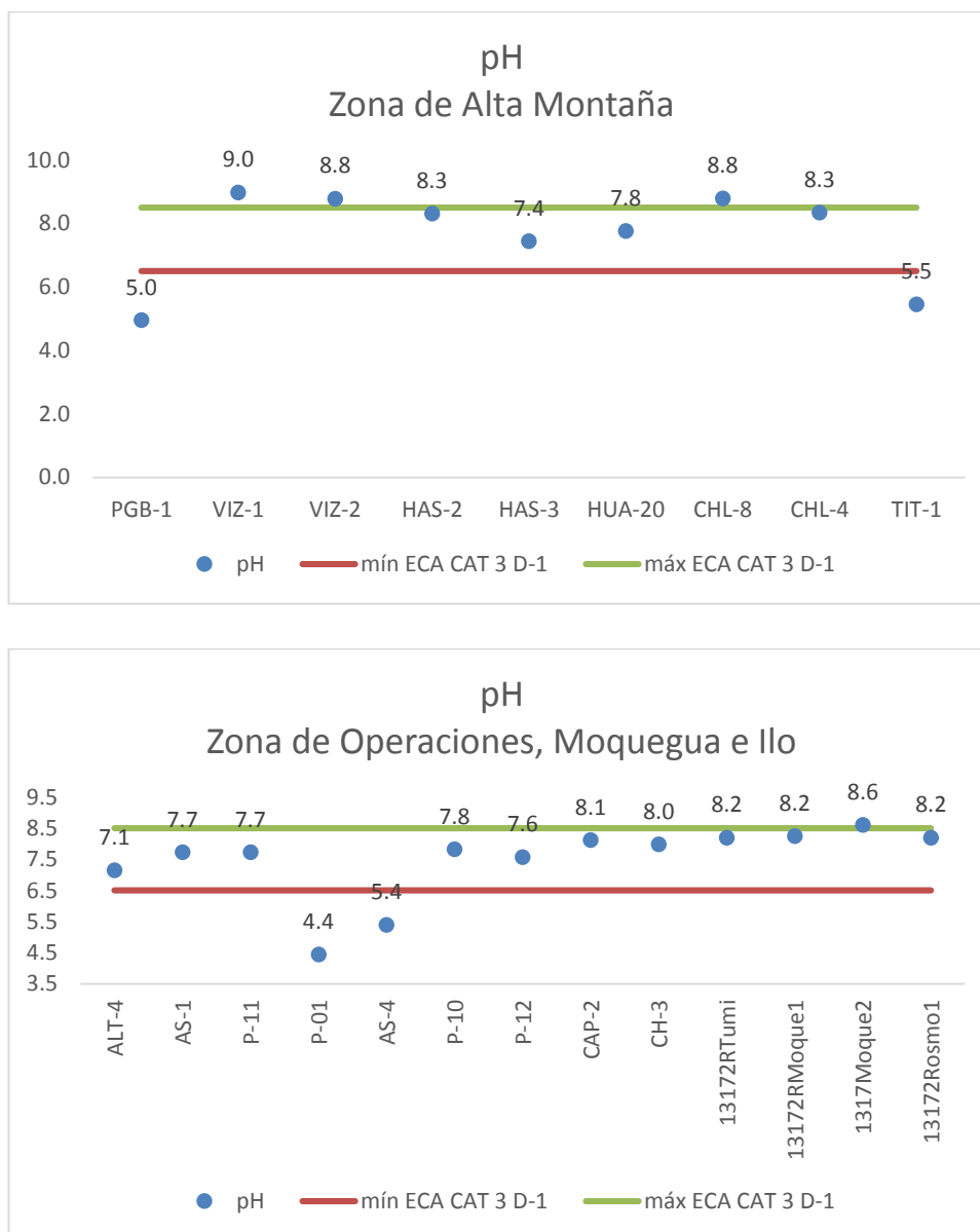
Gráfico 04. Variación Espacial del valor del pH de las estaciones de monitoreo de calidad de agua superficial – zona de alta montaña, zona de operaciones, Moquegua e Ilo del MAP-5 setiembre 2017.
