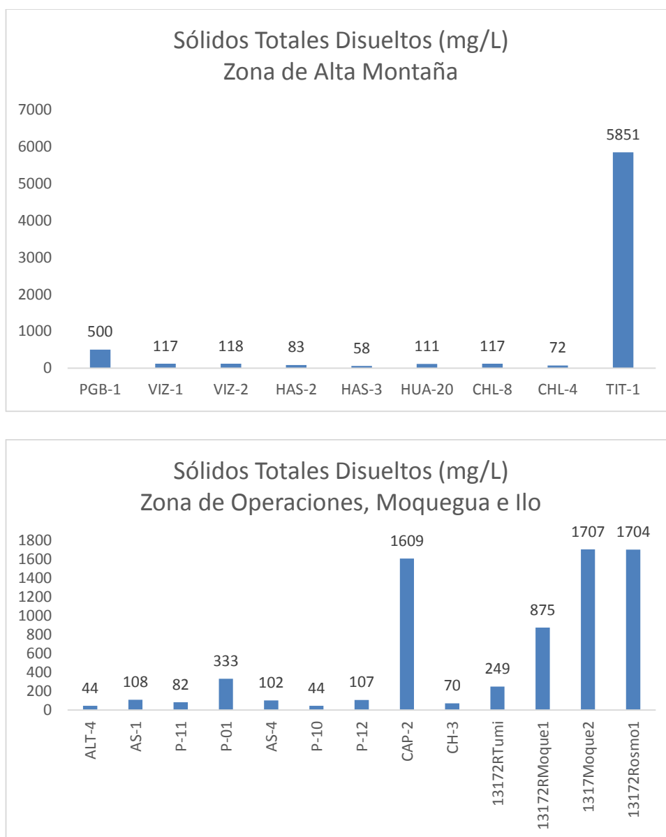
Gráfico 13. Variación espacial del contenido de sólidos totales disueltos de las diferentes estaciones de monitoreo de calidad de agua superficial – zona de alta montaña, zona de operaciones, Moquegua e Ilo del MAP-5 setiembre 2017.
