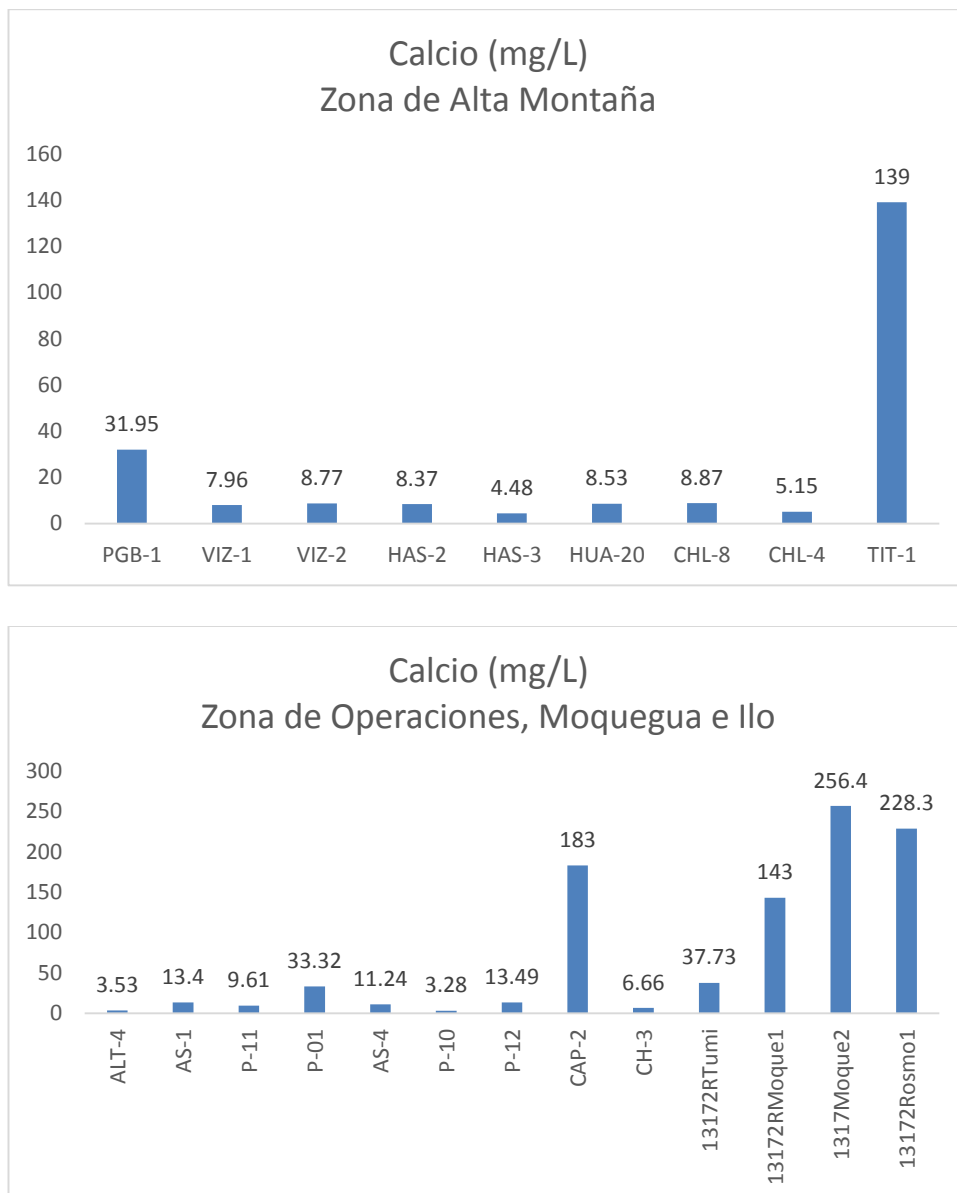
Gráfico 25. Variación espacial del contenido de calcio de las diferentes estaciones de monitoreo de calidad de agua superficial - zona de alta montaña, zona de operaciones, Moquegua e Ilo del MAP-5 setiembre 2017.
