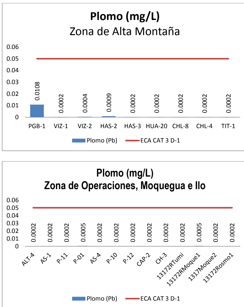
Gráfico 30. Variación espacial del contenido de plomo de las diferentes estaciones de monitoreo de calidad de agua superficial - zona de alta montaña, zona de operaciones, Moquegua e Ilo del MAP-5 setiembre 2017.
