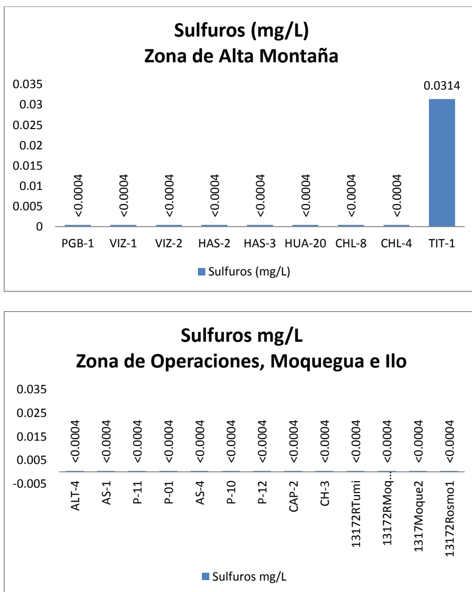
Gráfico 15. Variación espacial del contenido de sulfuros de las diferentes estaciones de monitoreo de calidad de agua superficial – zona de alta montaña, zona de operaciones, Moquegua e Ilo del MAP-5 setiembre 2017.
