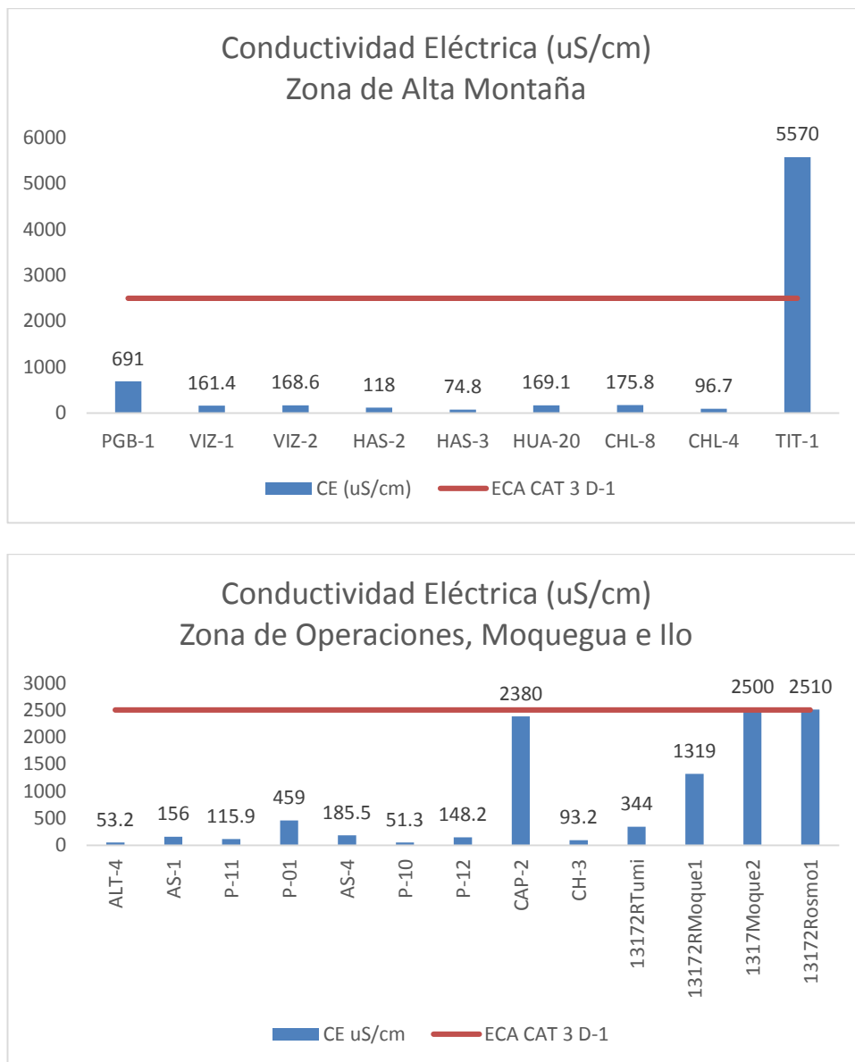
Gráfico 05. Variación espacial del valor de la conductividad de las diferentes estaciones de monitoreo de calidad de agua superficial – zona de alta montaña, zona de operaciones, Moquegua e Ilo del MAP-5 setiembre 2017.
