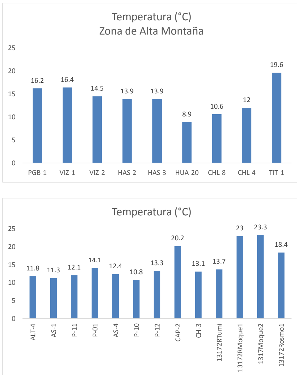
Gráfico 02. Variación espacial de la temperatura de las estaciones de monitoreo de calidad de agua superficial – zona de alta montaña, zona de operaciones, Moquegua e Ilo del MAP-5 setiembre 2017.
