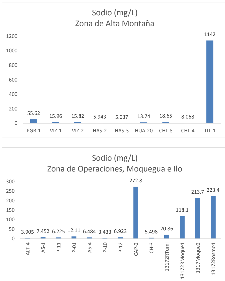
Gráfico 31. Variación espacial del contenido de sodio de las diferentes estaciones de monitoreo de calidad de agua superficial - zona de alta montaña, zona de operaciones, Moquegua e Ilo del MAP-5 setiembre 2017.
