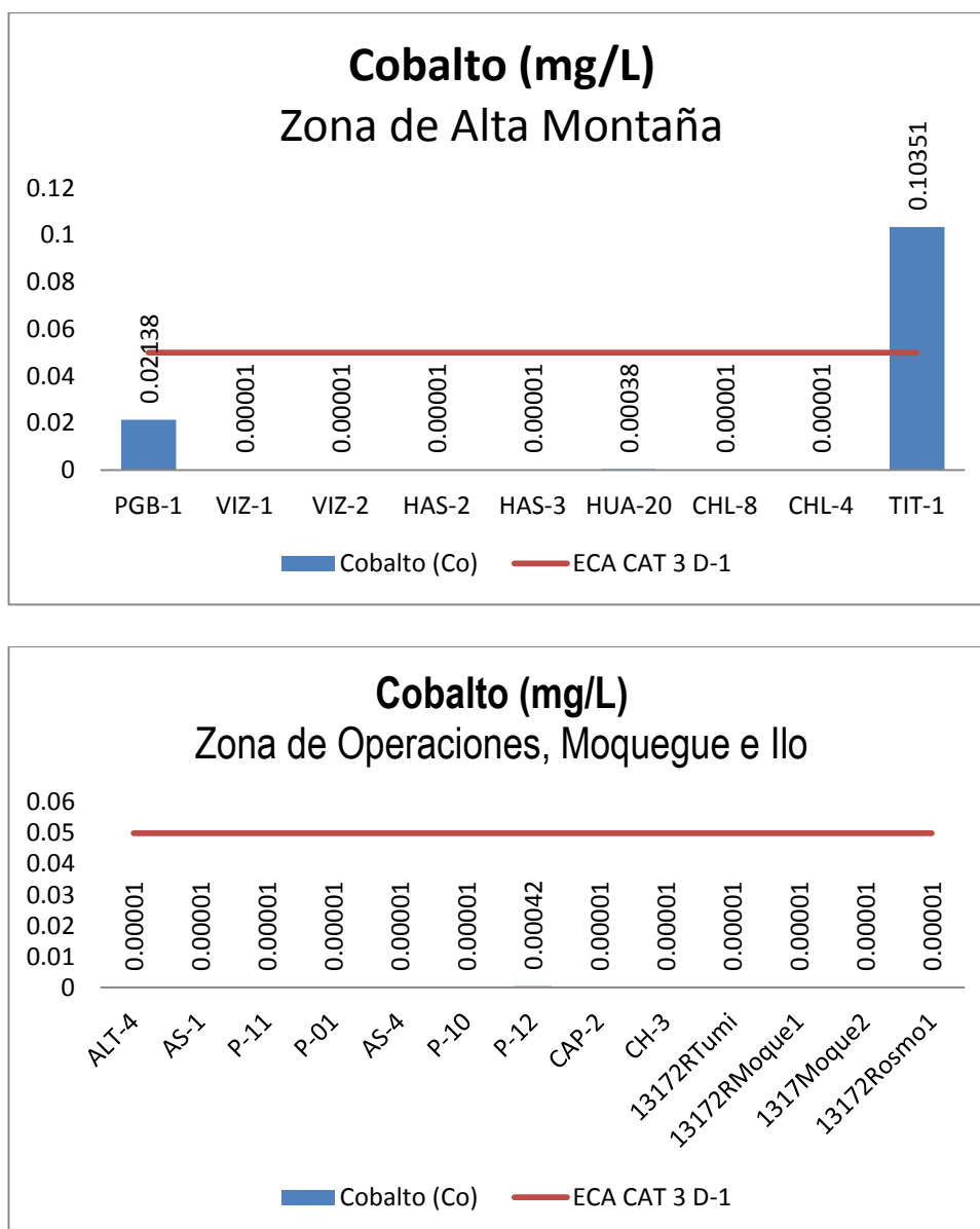
Gráfico 26. Variación espacial del contenido de cobalto de las diferentes estaciones de monitoreo de calidad de agua superficial - zona de alta montaña, zona de operaciones, Moquegua e Ilo del MAP-5 setiembre 2017.
