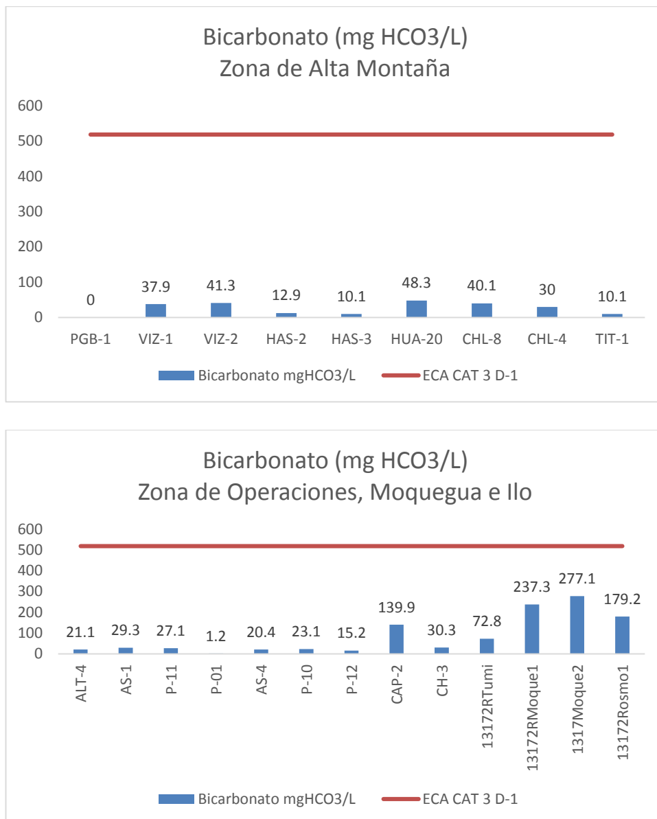
Gráfico 07. Variación espacial del valor del contenido de bicarbonato de las diferentes estaciones de monitoreo de calidad de agua superficial – zona de alta montaña, zona de operaciones, Moquegua e Ilo del MAP-5 setiembre 2017.
