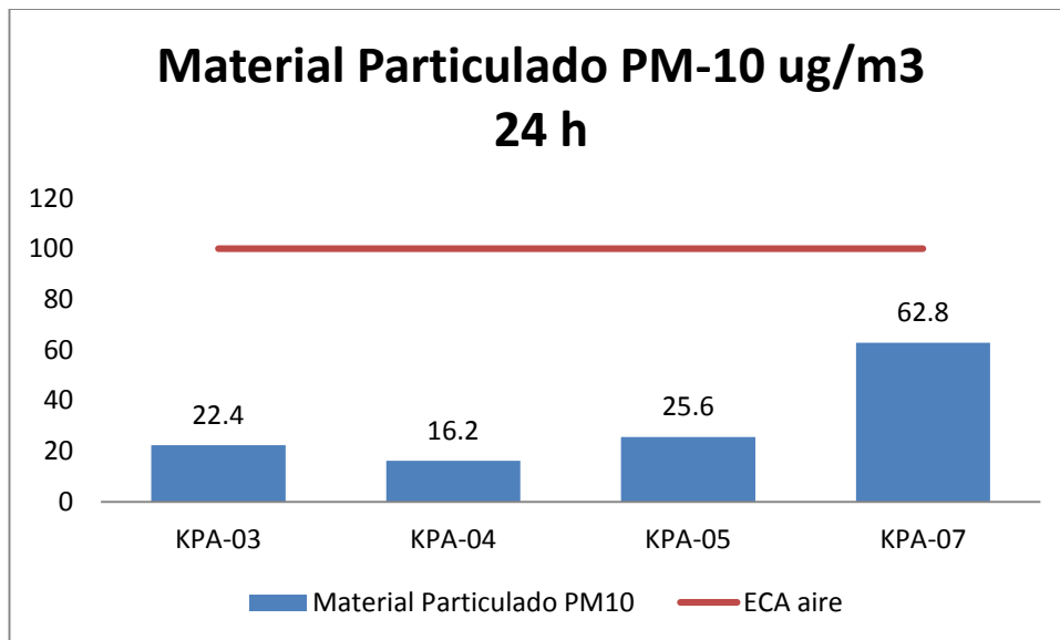
Gráfico 37. Variación espacial del contenido de material particulado menor a 10 \mu\text{m} de las diferentes estaciones de monitoreo de calidad de aire del MAP-5 setiembre 2017.
