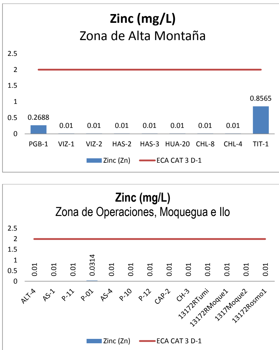
Gráfico 32. Variación espacial del contenido de Zinc de las diferentes estaciones de monitoreo de calidad de agua superficial - zona de alta montaña, zona de operaciones, Moquegua e Ilo del MAP-5 setiembre 2017.
