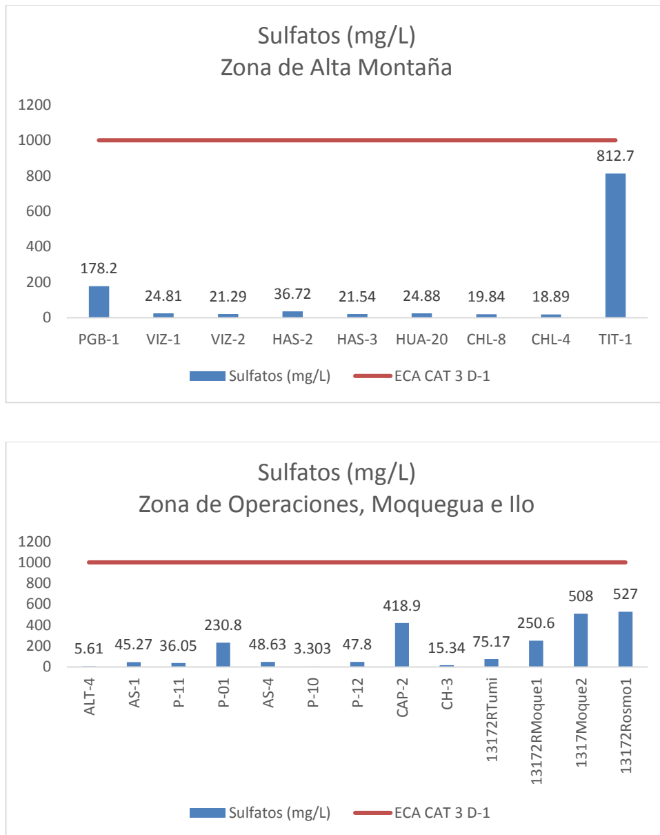
Gráfico 19. Variación espacial del contenido de sulfatos en las estaciones de monitoreo de calidad de agua superficial - zona de alta montaña, zona de operaciones, Moquegua e Ilo del MAP-5 setiembre 2017.
