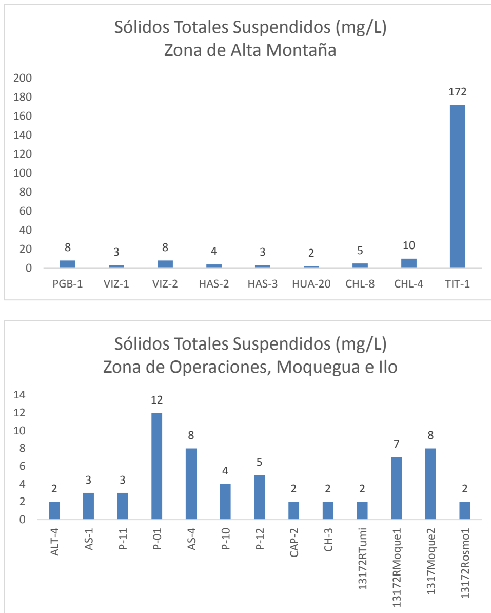
Gráfico 14. Variación espacial del contenido de sólidos totales en suspensión de las diferentes estaciones de monitoreo de calidad de agua superficial – zona de alta montaña, zona de operaciones, Moquegua e Ilo del MAP-5 setiembre 2017.
