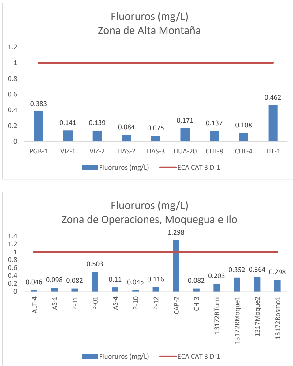
Gráfico 17. Variación espacial del contenido de fluoruros de las estaciones de monitoreo de calidad de agua superficial - zona de alta montaña, zona de operaciones, Moquegua e Ilo del MAP-5 setiembre 2017.
