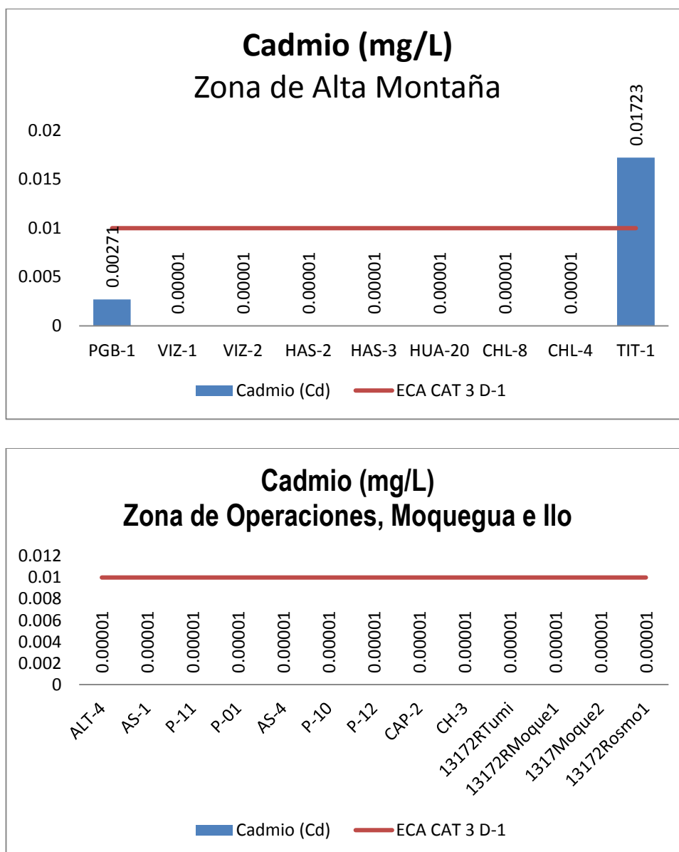
Gráfico 24. Variación espacial del contenido de cadmio de las diferentes estaciones de monitoreo de calidad de agua superficial - zona de alta montaña, zona de operaciones, Moquegua e Ilo del MAP-5 setiembre 2017.
