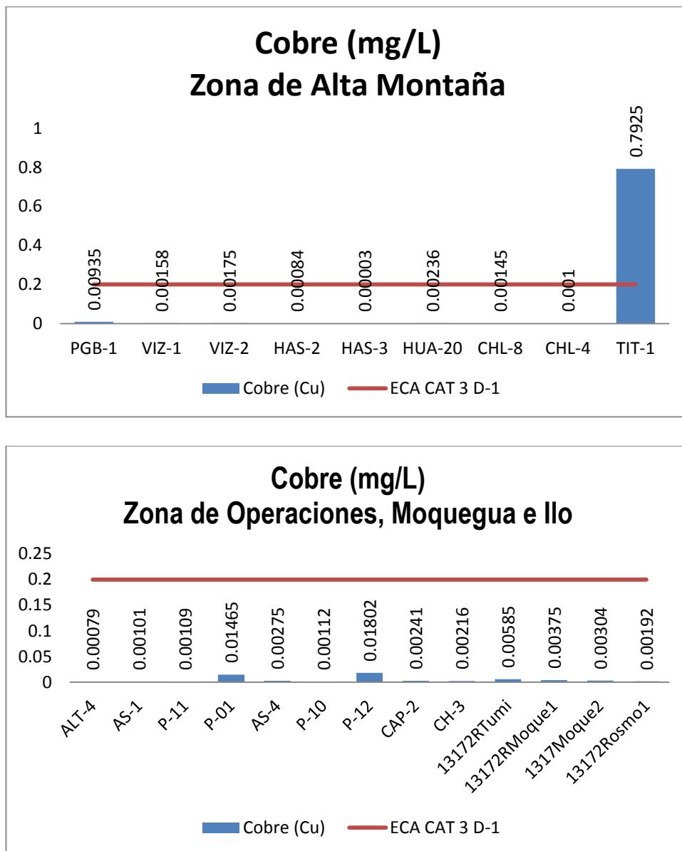
Gráfico 27. Variación espacial del contenido de cobre en las estaciones de monitoreo de calidad de agua superficial - zona de alta montaña, zona de operaciones, Moquegua e Ilo del MAP-5 setiembre 2017.
