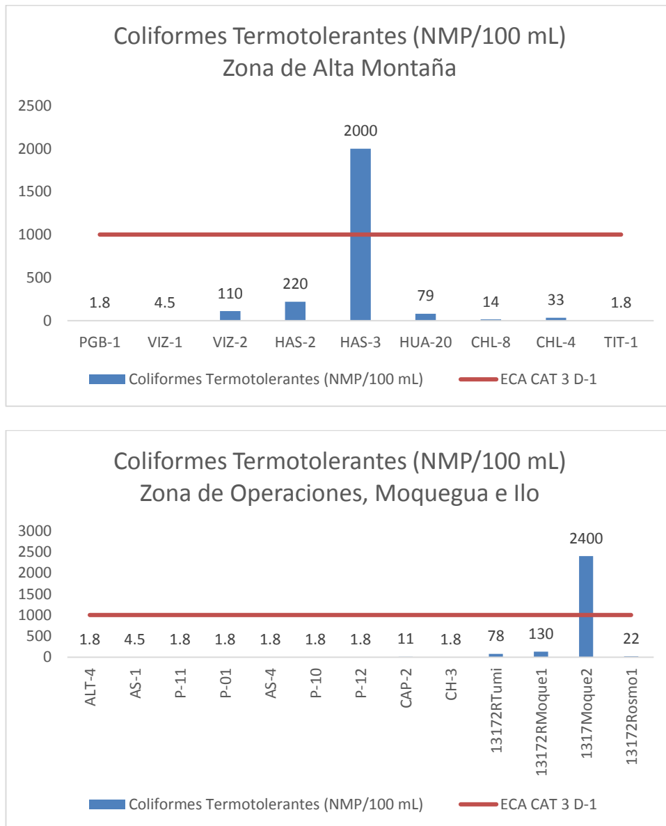
Gráfico 33. Variación espacial de la numeración de fecales de las diferentes estaciones de monitoreo de calidad de agua superficial - zona de alta montaña, zona de operaciones, Moquegua e Ilo del MAP-5 setiembre 2017.
